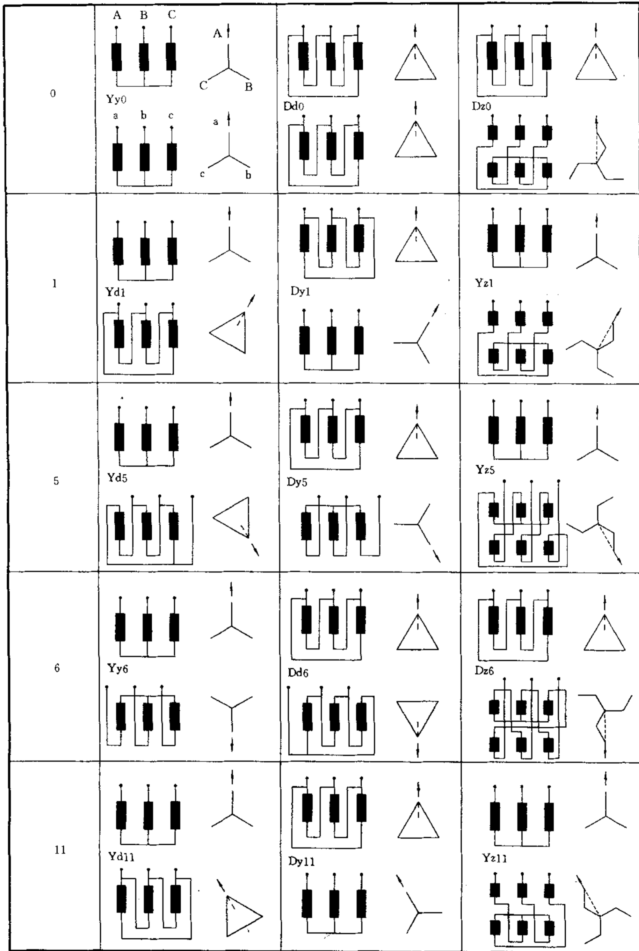
图 D1 常用的联结组
