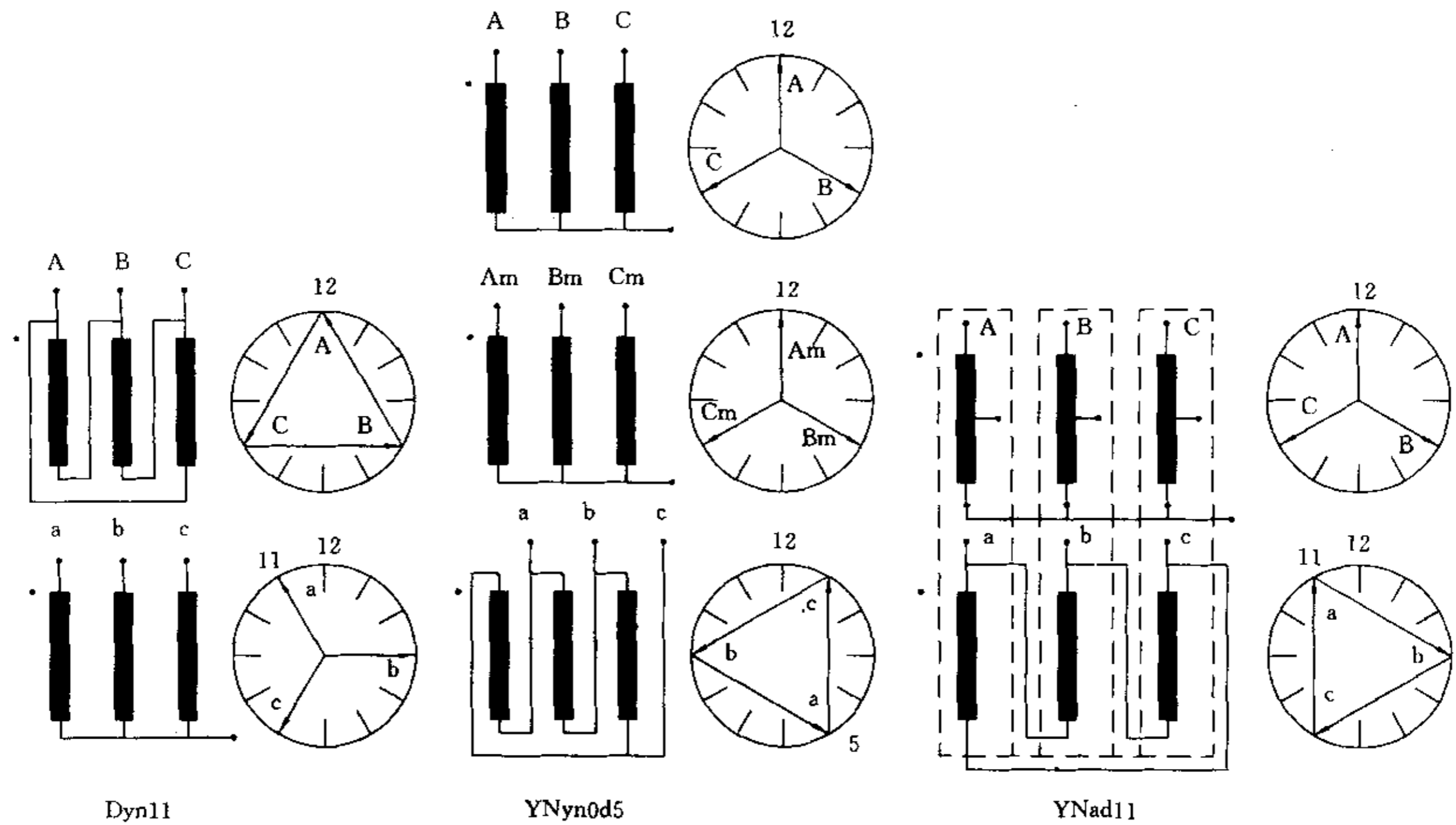
图 2 钟时序数表示法(三个例子)
