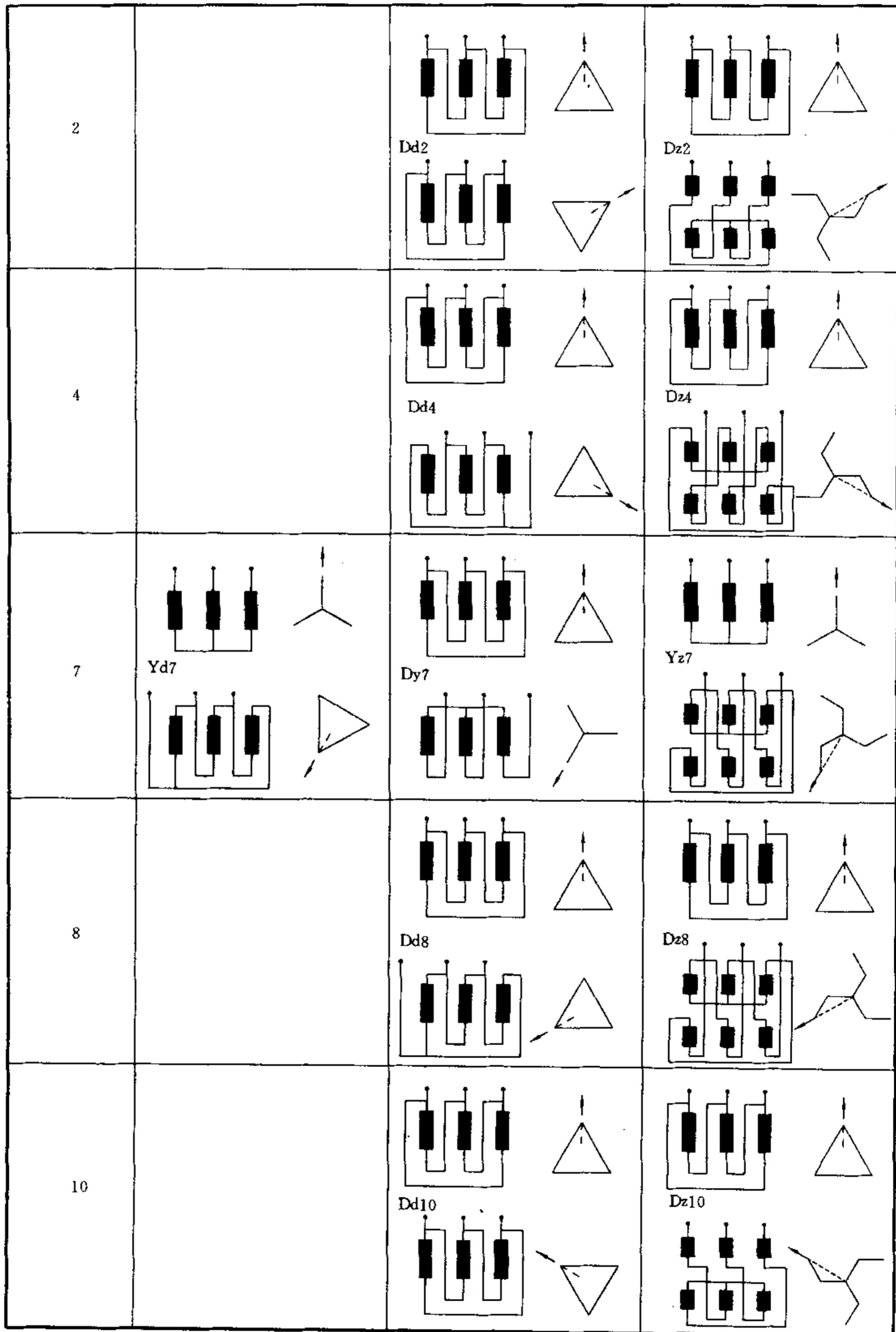
图 D2 补充的联结组
