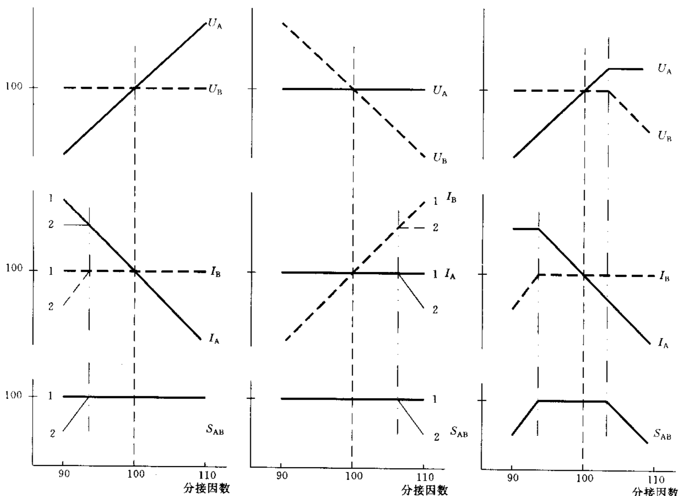
图 1a 恒磁通调压
