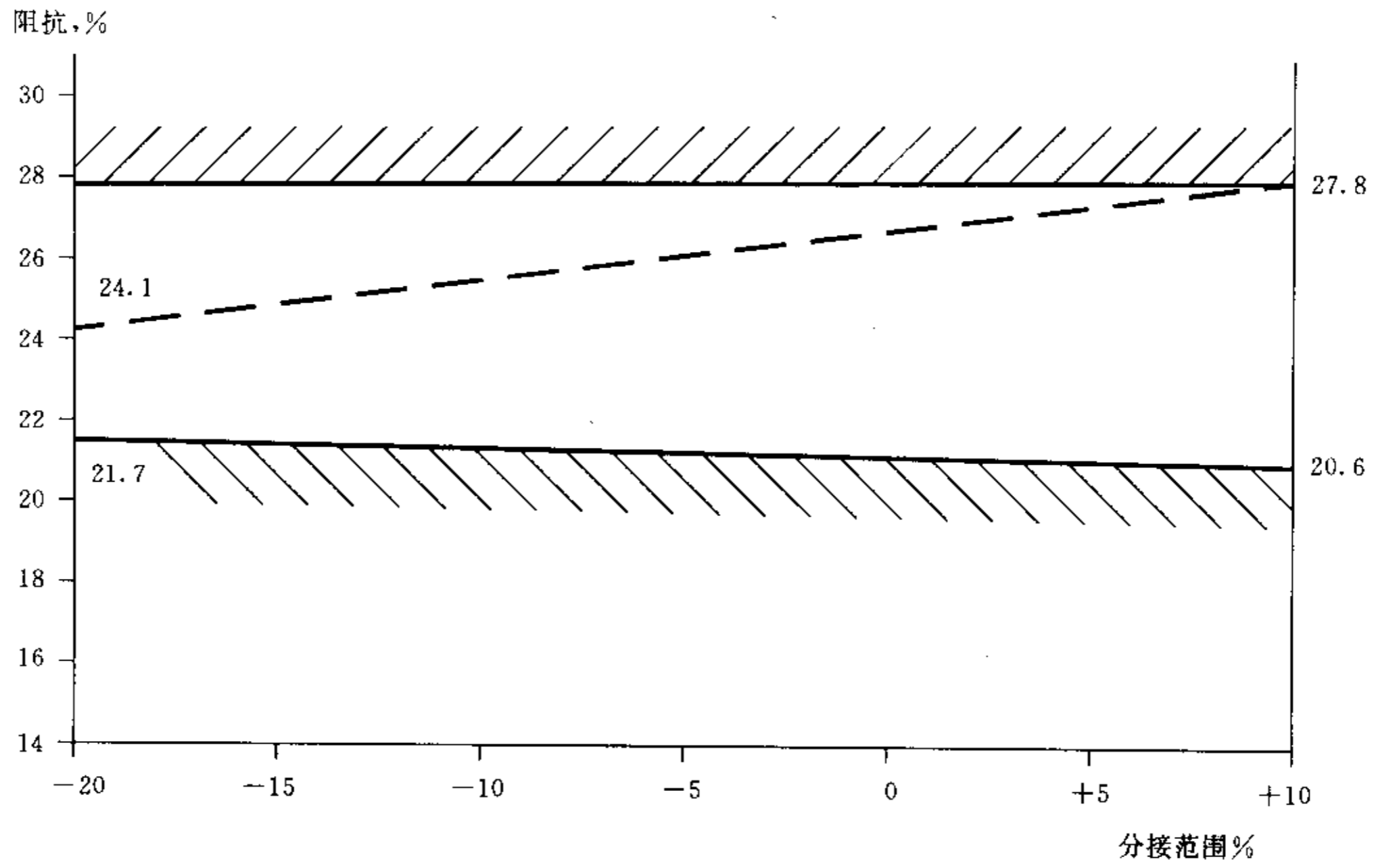
图 C1 用界限法表示短路阻抗规范的举例
