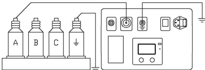
图 3 无串联间隙过电压保护器试验接线图
